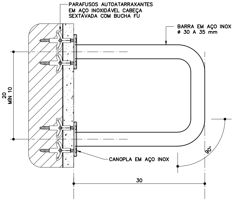
DETALHE 2 ESC. 1:5
