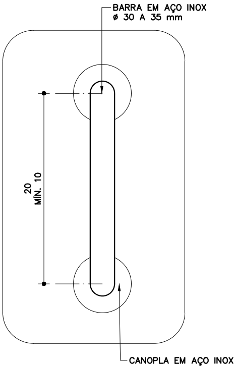
DETALHE 01 ESC. 1:5
