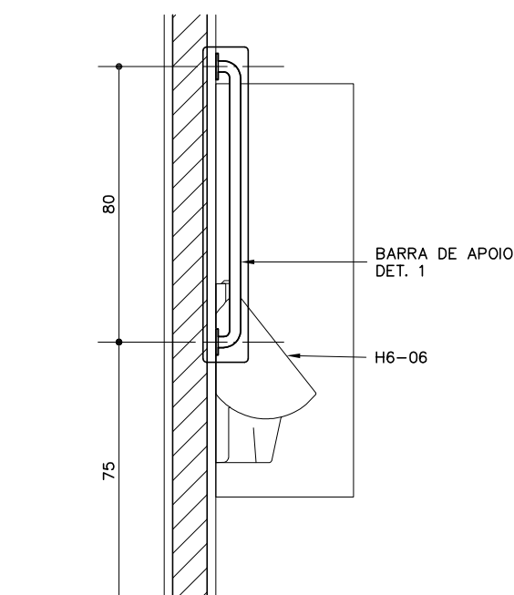
CORTE AA
