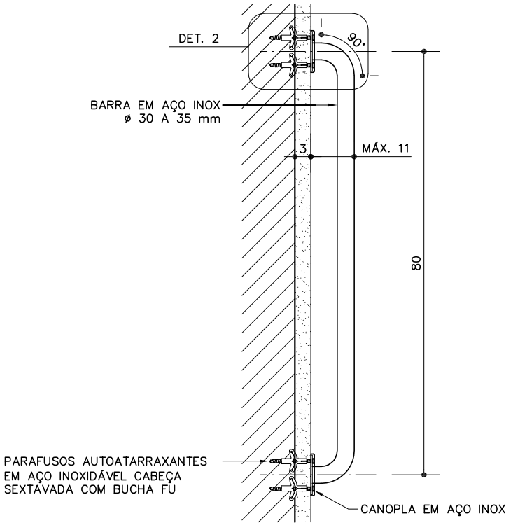
DETALHE 1. BARRA DE APOIO ESC. 1:10
