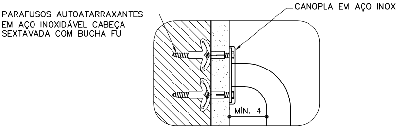
DETALHE 2 ESC. 1:5
