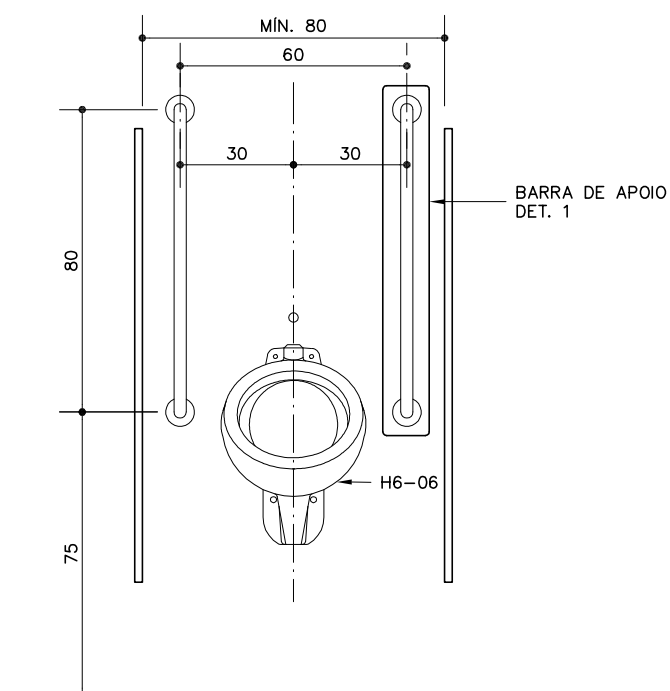
VISTA
