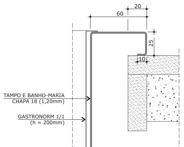
DETALHE 1 ESC. 1:2,5
