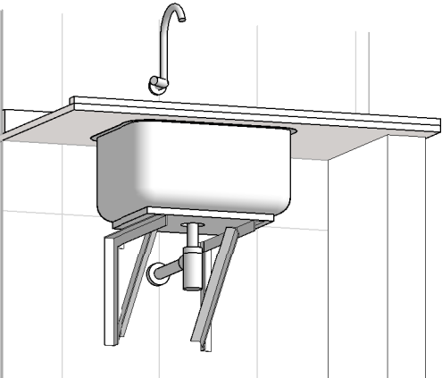
SUPORTE METÁLICO
