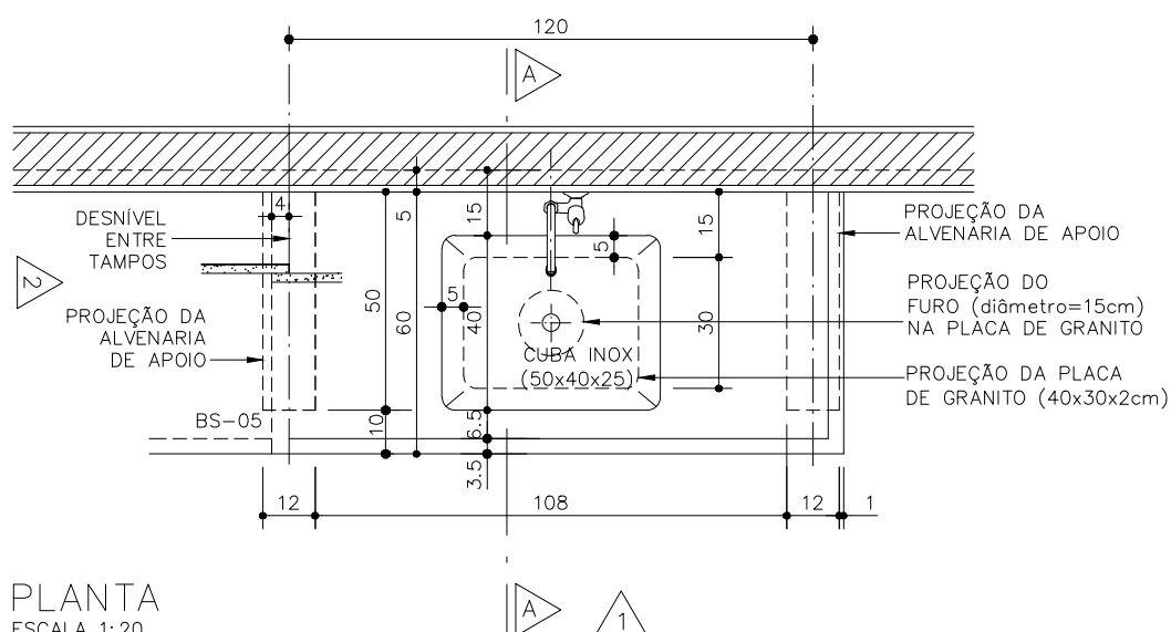
EXEMPLO DE COMPOSIÇÃO CC-03 E BS-05
