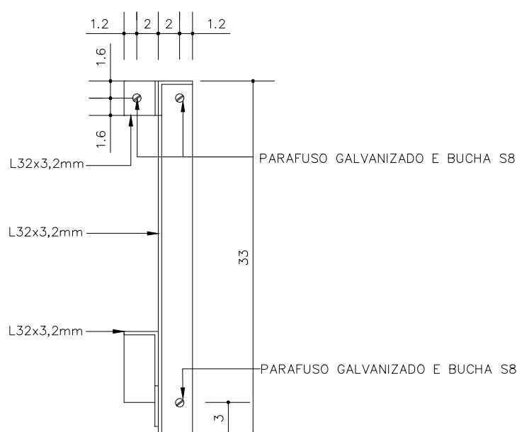
CORTE BB ESCALA 1:5
