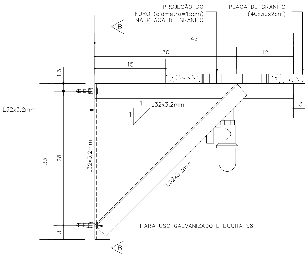
VISTA 2 ESCALA 1:5
