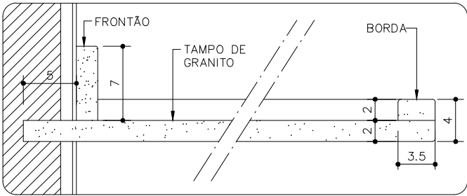
DETALHE 1 ESCALA 1:5
