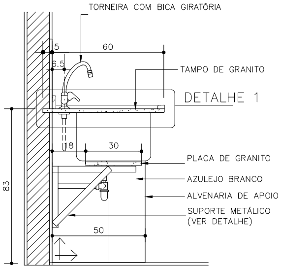
CORTE AA ESCALA 1:20
