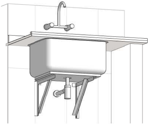
SUPORTE METÁLICO
