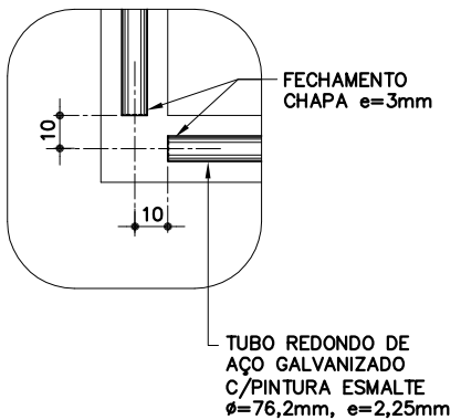
AMPLIAÇÃO 1 ESC. 1:25
