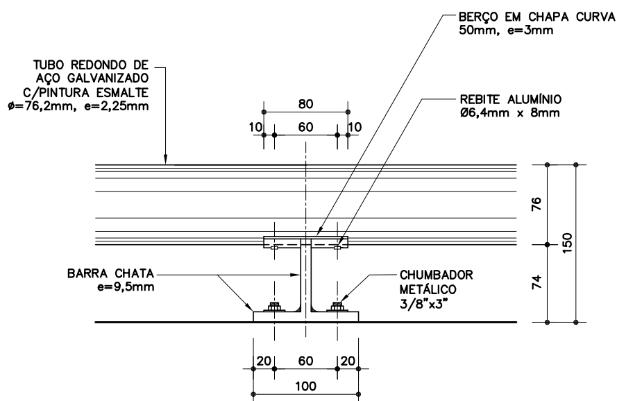
VISTA ESC. 1:5
