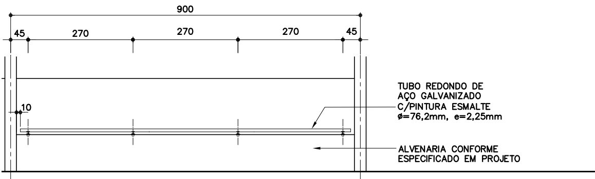
EXEMPLO 3 ESC. 1:100
