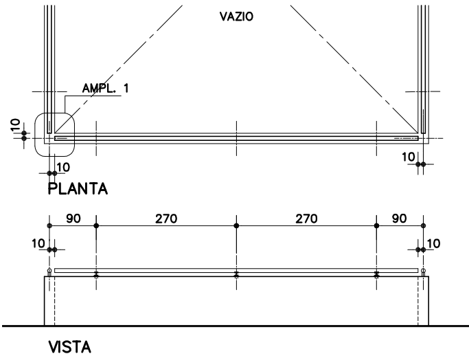
EXEMPLO 4 ESC. 1:100
