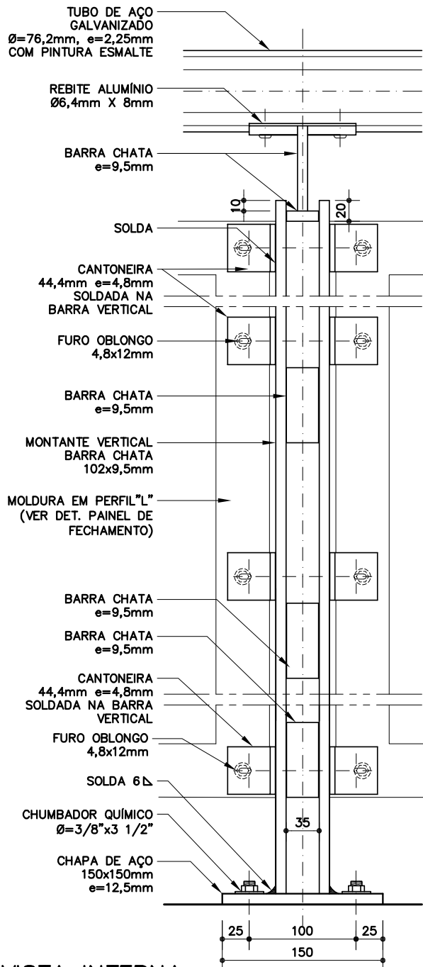
VISTA INTERNA
