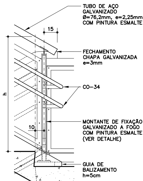
AMPL. 8 ESC. 1:25
