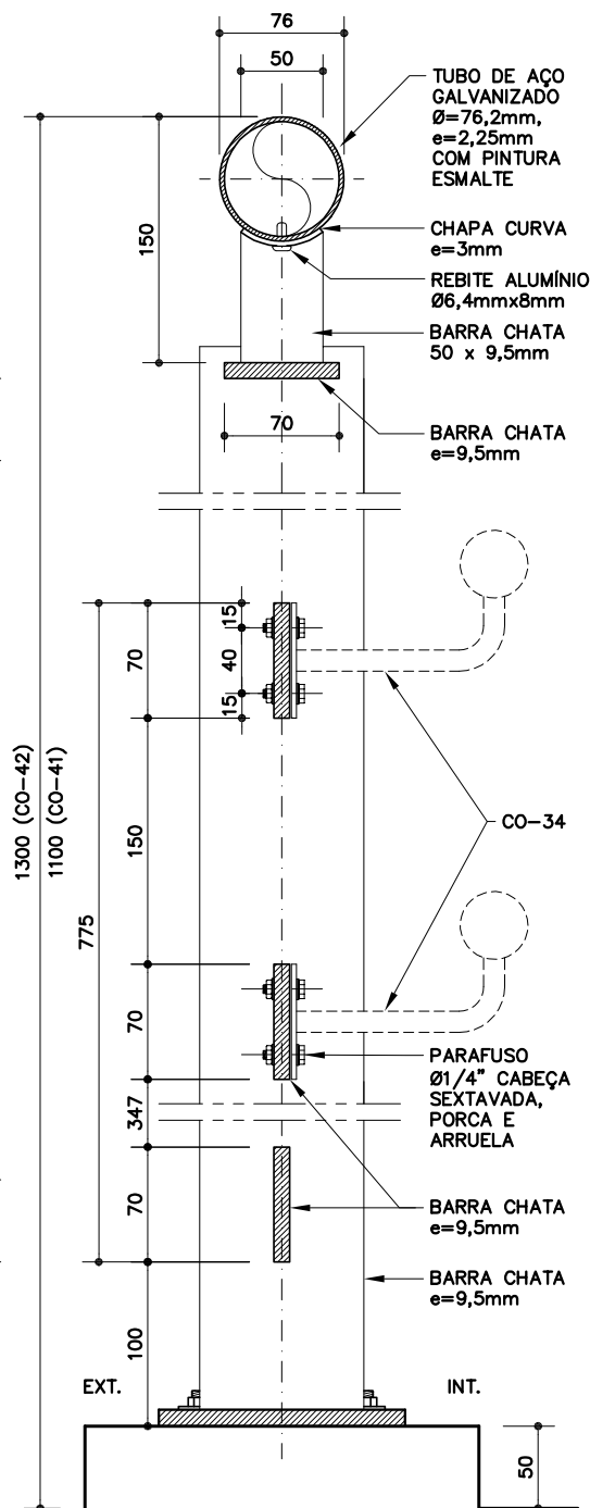
CORTE TRANSVERSAL
