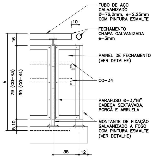
AMPL. 9 ESC. 1:25
