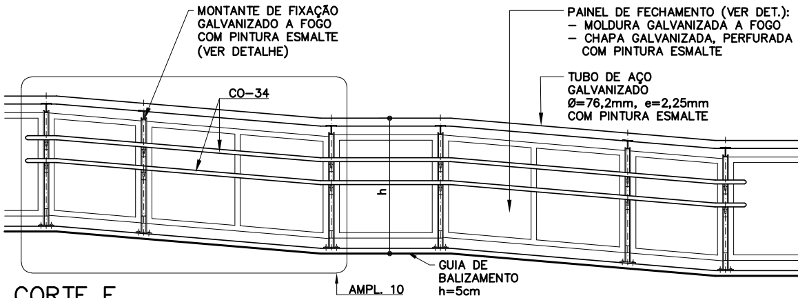
CORTE E ESC. 1: 50
