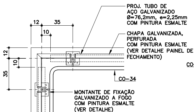
AMPL. 1 ESC. 1:25
