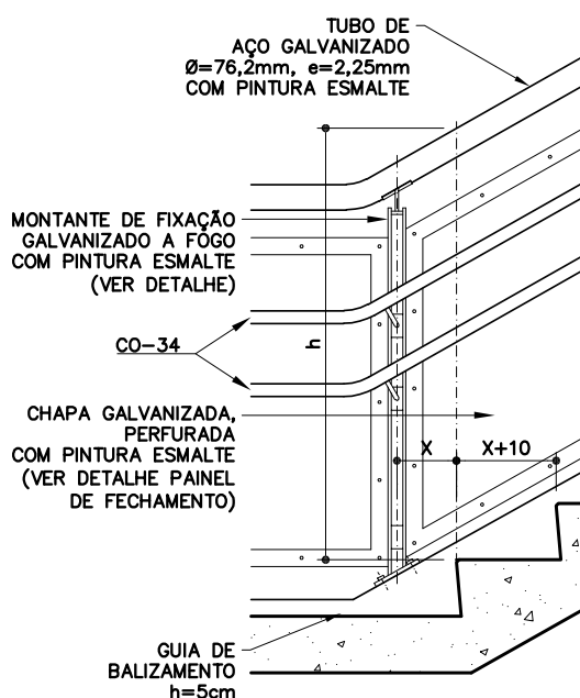
AMPL. 3 ESC. 1:25
