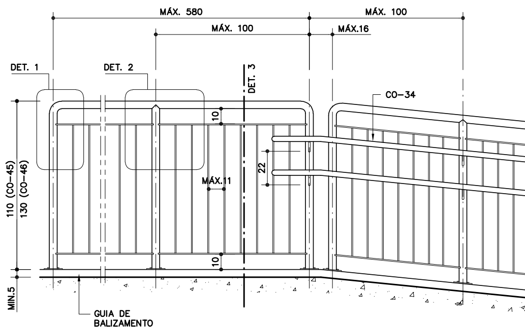
VISTA GENÉRICA - RAMPA ESC. 1:25
