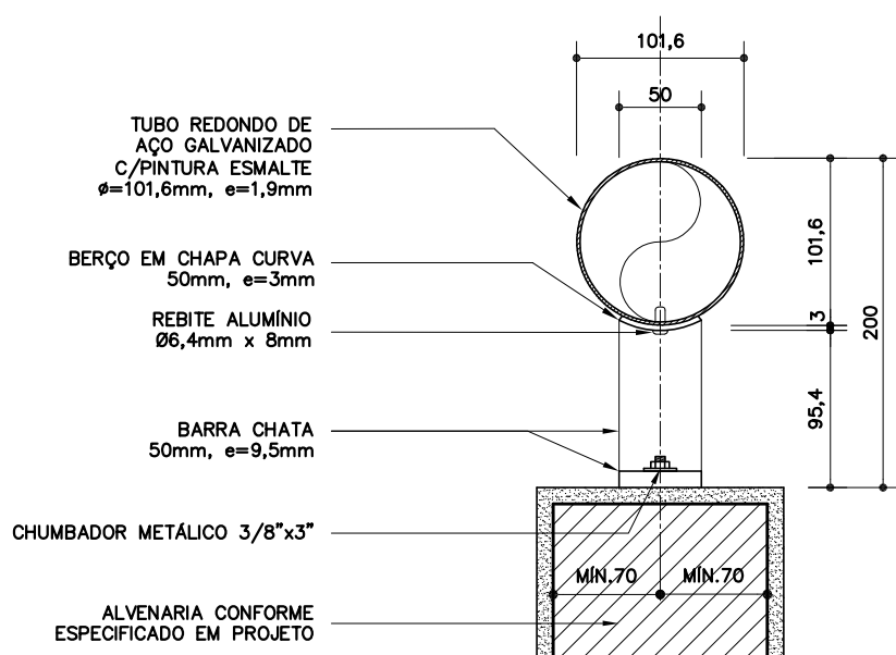
CORTE TRANSVERSAL ESC. 1:5
