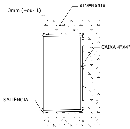
DETALHE DA CAIXA 4"x4" ESC. 1:2
