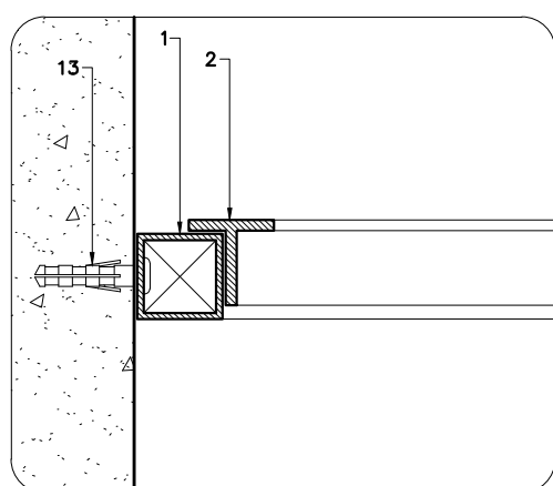
DET. 3 ESC. 1:2,5
