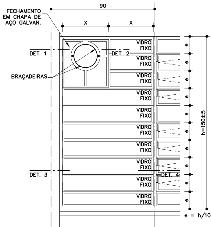
VISTA EXTERNA ESC. 1:20
