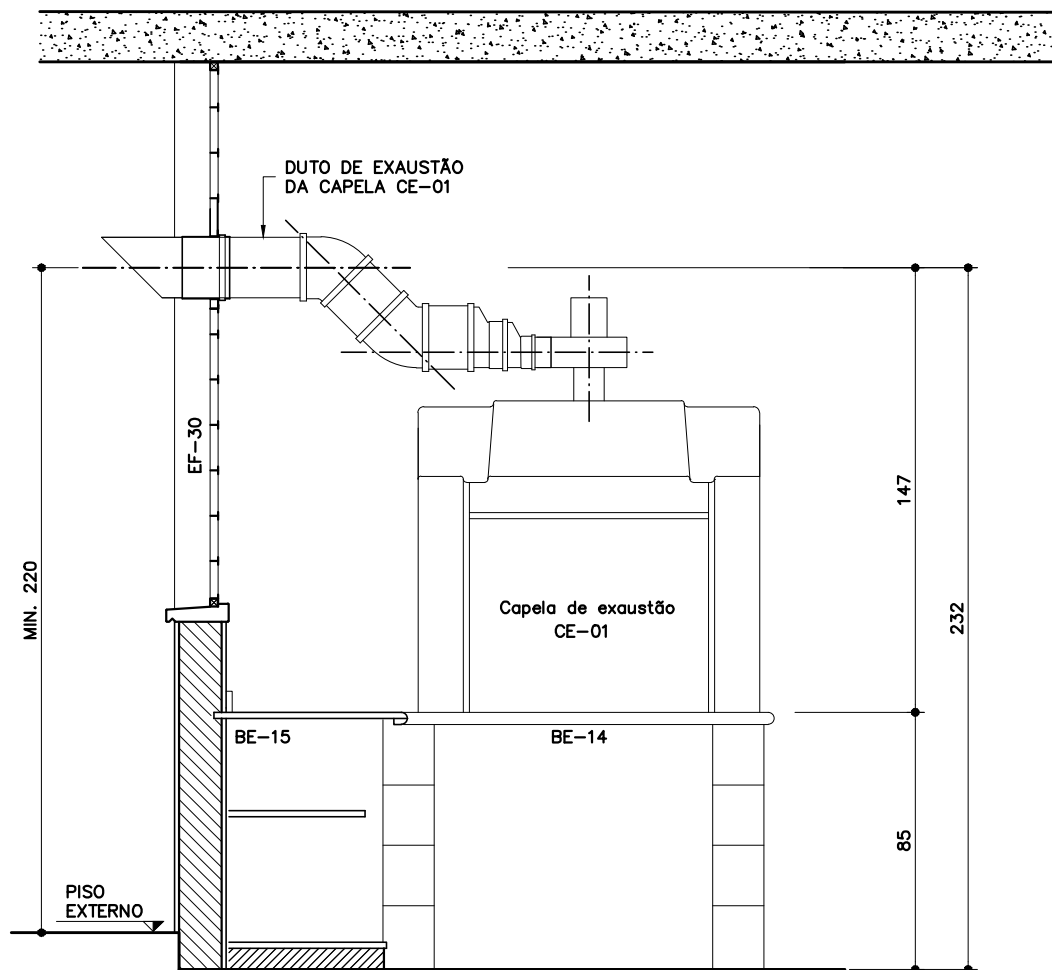
VISTA ESC. 1:25
