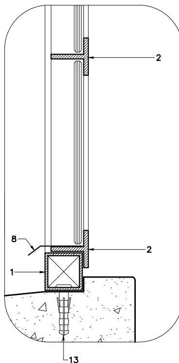
DET. 6 ESC. 1:2,5
