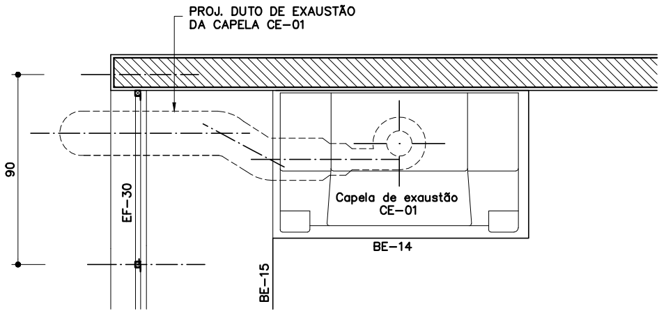
PLANTA ESC. 1:25
