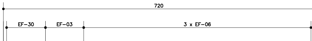
PLANTA ESC. 1:20
