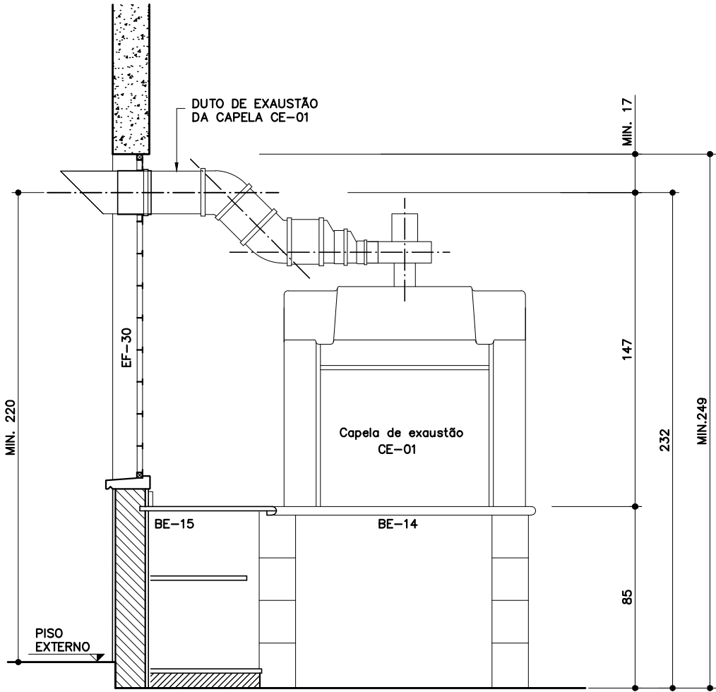
VISTA ESC. 1:25
