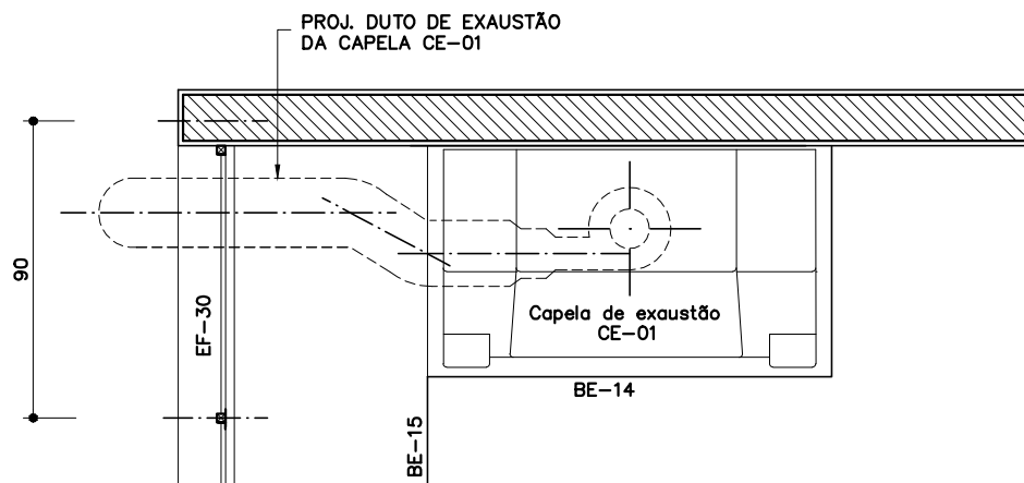
PLANTA ESC. 1:25
