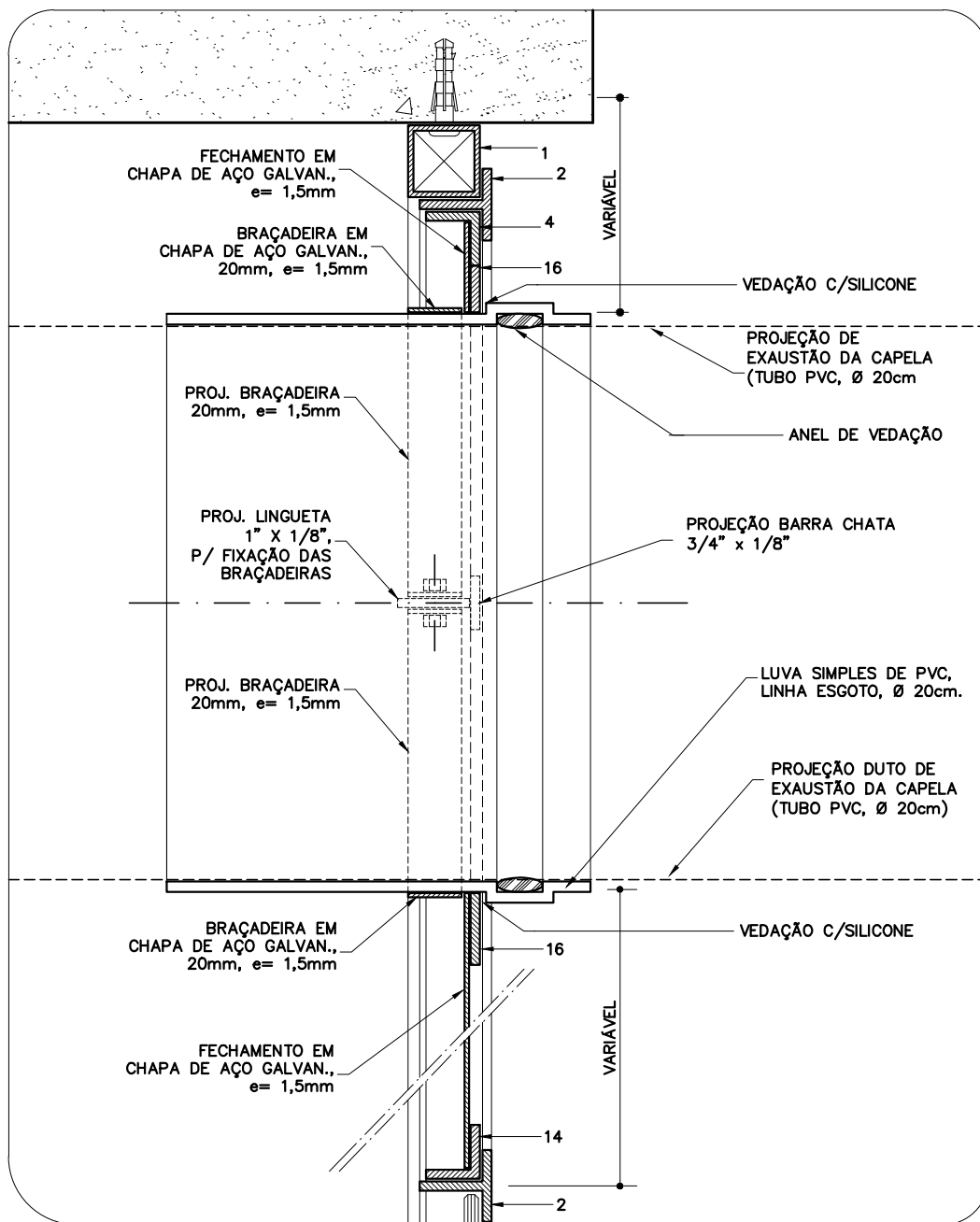
DET. 5 ESC. 1:2,5
