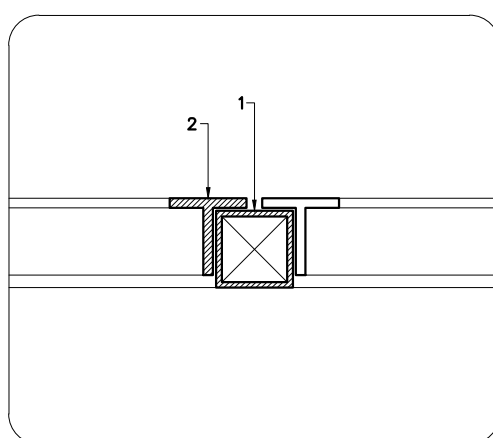
DET. 4 ESC. 1:2,5
