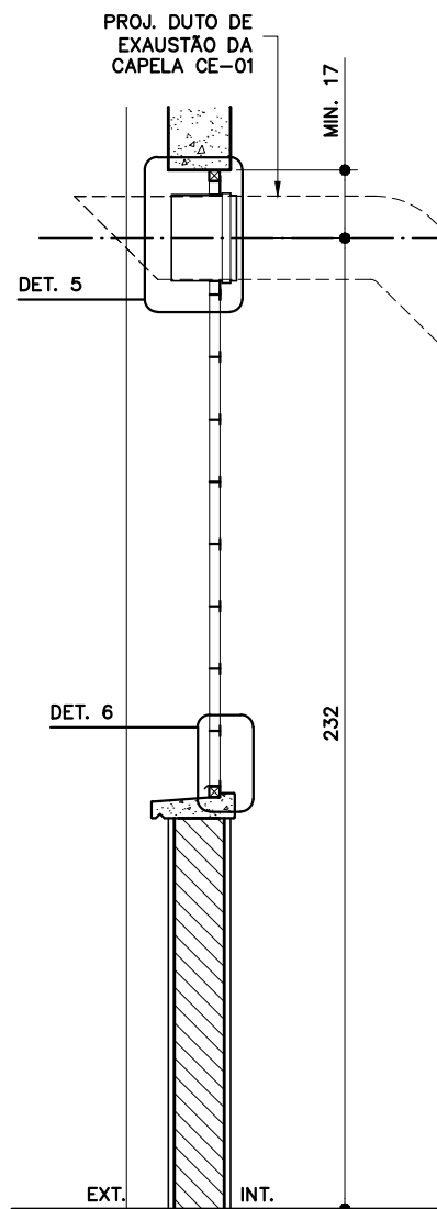
CORTE AA ESC. 1:20
