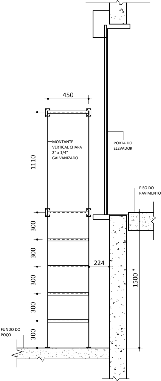
CORTE AA ESC: 1 : 25
