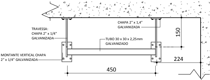
DETALHE ESC: 1 : 10
