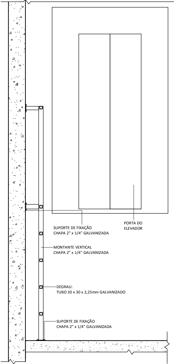
CORTE BB ESC: 1 : 25
