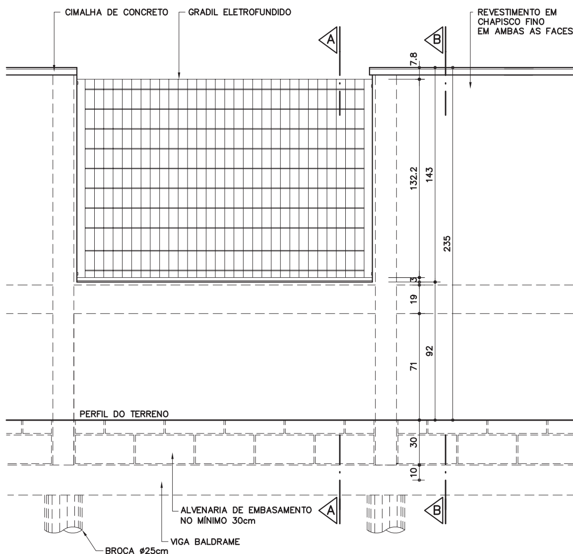
VISTA 1 ESC. 1: 25
