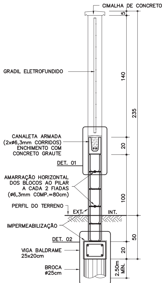
CORTE AA ESC. 1:25
