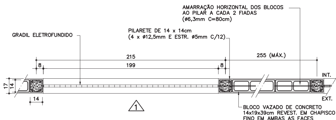
PLANTA ESC. 1: 25
