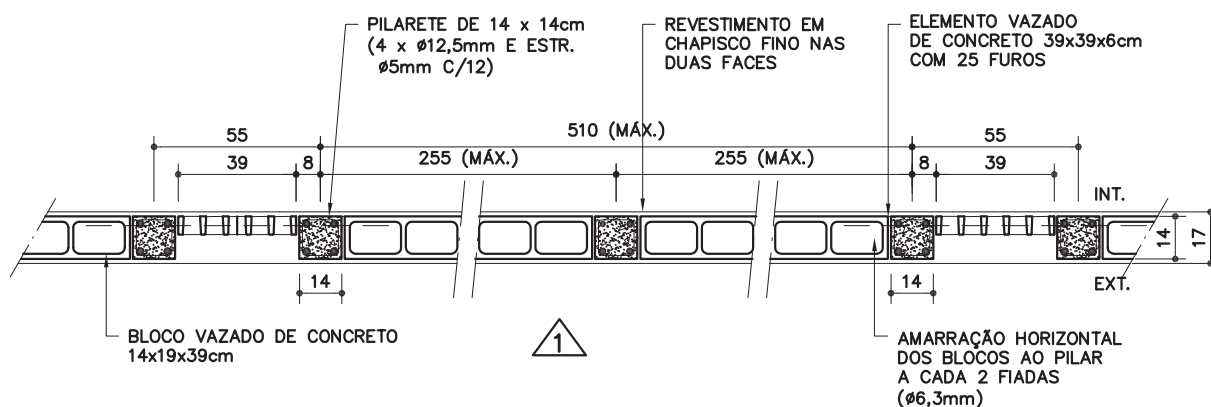
PLANTA ESC. 1:25
