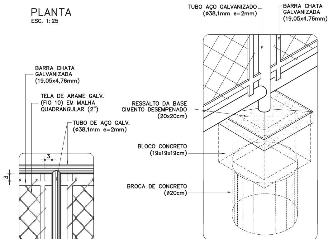
DETALHE 1 ESC. 1:10
