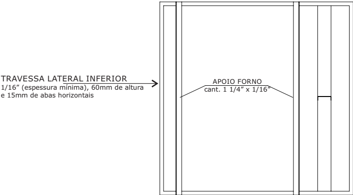
TRAVESSAS INFERIORES
