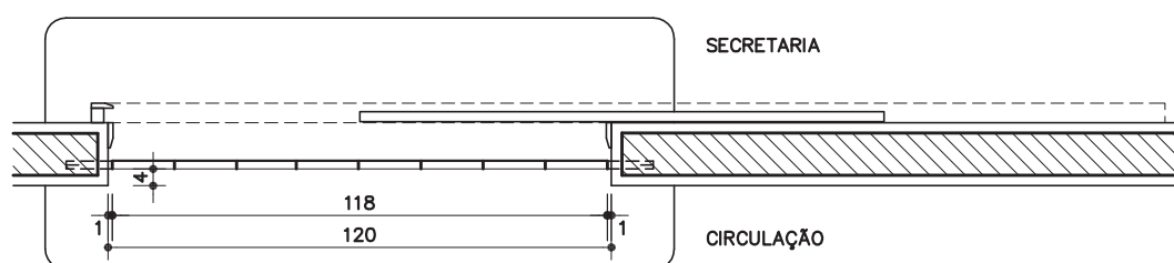
PLANTA GR-02 COM GS-04 ESC. 1:20
