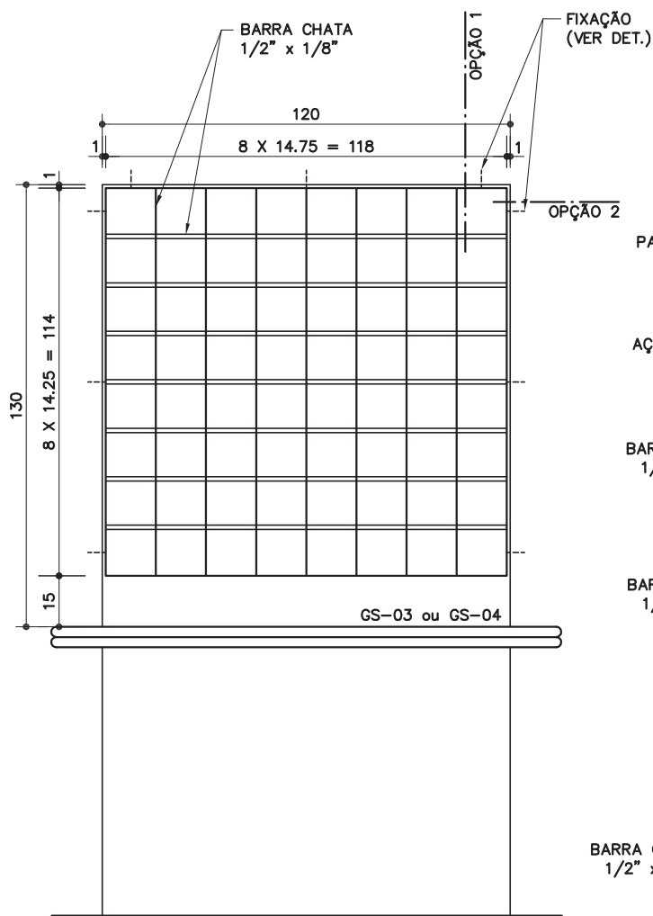
VISTA DA CIRCULAÇÃO ESC. 1:20
