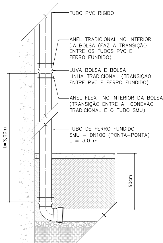
TUBULAÇÃO SOB LEITO CARROÇÁVEL S/ESC.
