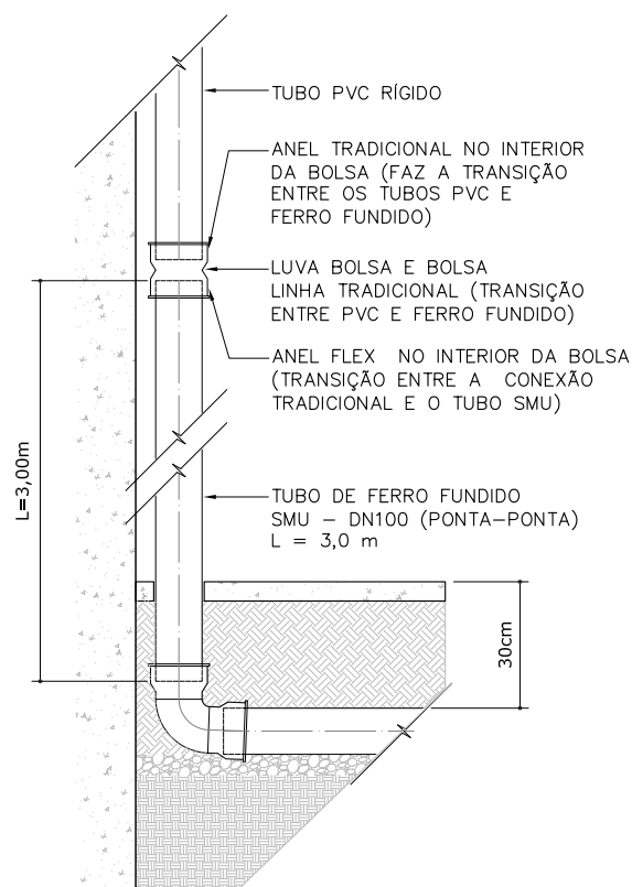
TUBULAÇÃO SOB VIAS DE PEDESTRES S/ESC.
