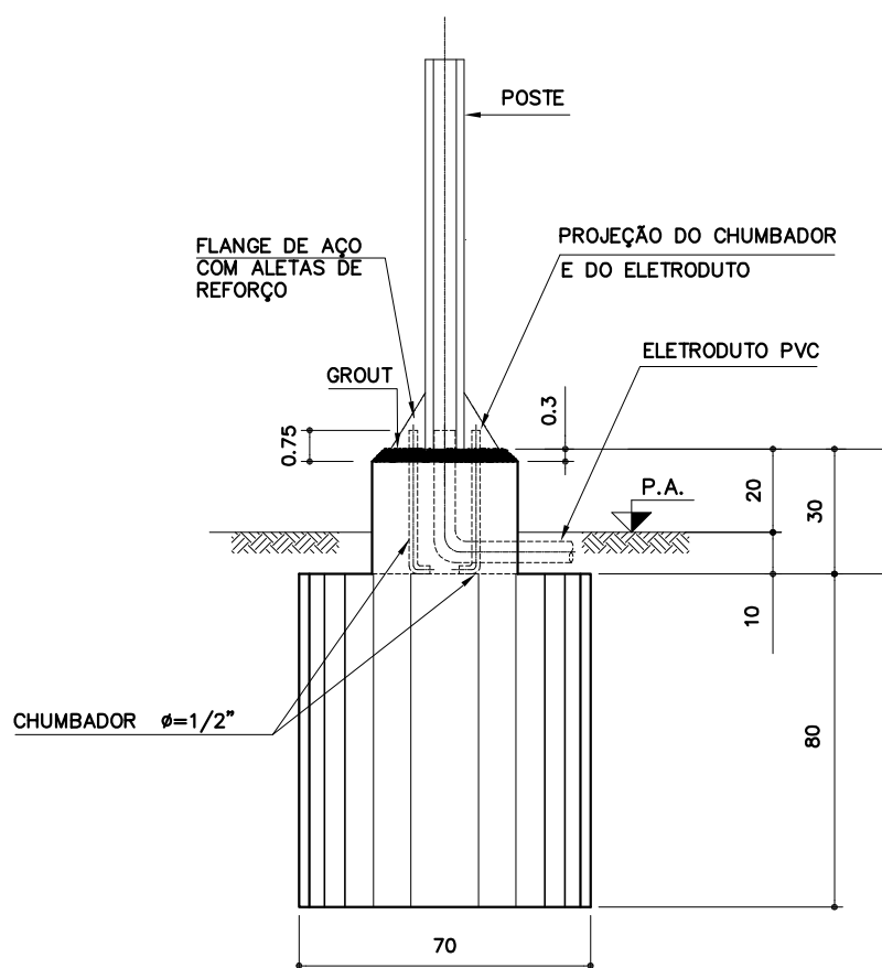
CORTE AA
