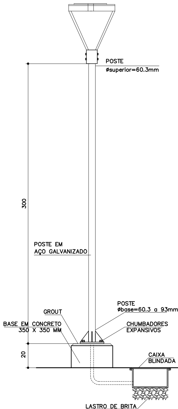
VISTA S/ESC.
