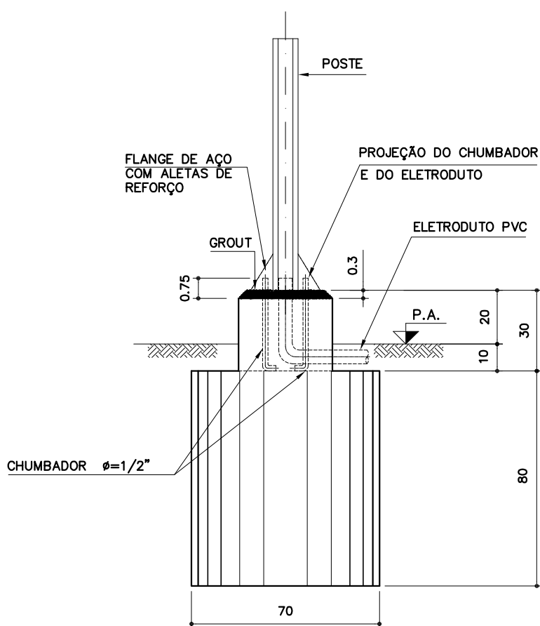
CORTE AA
