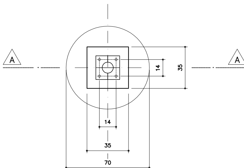
PLANTA
