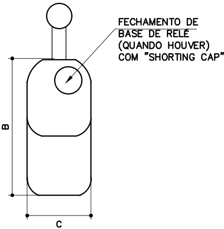
VISTA SUPERIOR S/ESC.
