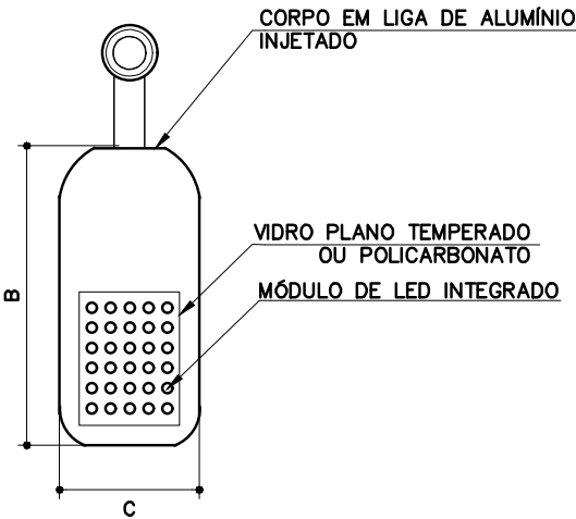
VISTA INFERIOR S/ESC.
