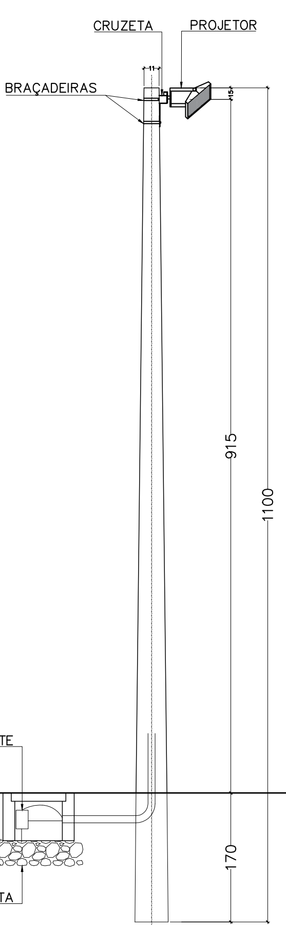
CORTE AA SEM ESCALA
