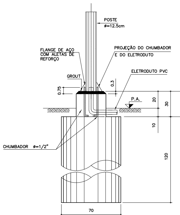
CORTE AA ESC.1: 20
