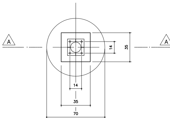
PLANTA ESC.1: 20
