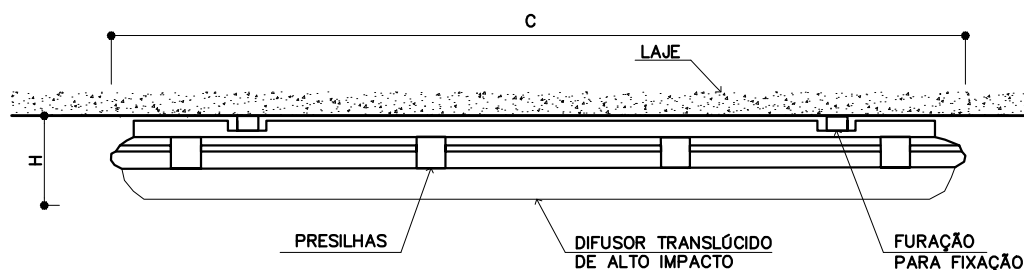
IL-86 LUMINÁRIA HERMÉTICA CORTE LONGITUDINAL S/ESC.
