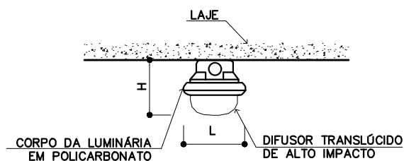
IL-86 LUMINÁRIA HERMÉTICA CORTE TRANSVERSAL S/ESC.
