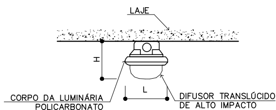
IL-87 LUMINÁRIA HERMÉTICA CORTE TRANSVERSAL S/ESC.
