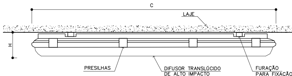
IL-87 LUMINÁRIA HERMÉTICA CORTE LONGITUDINAL S/ESC.
