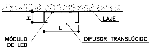
IL-88 LUMINÁRIA LED INTEGRADA CORTE TRANSVERSAL S/ESC.
