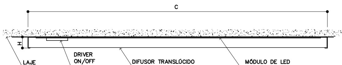
IL-88 LUMINÁRIA LED INTEGRADA CORTE LONGITUDINAL S/ESC.
