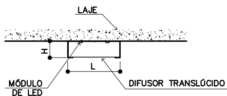
IL-90 LUMINÁRIA LED INTEGRADA CORTE TRANSVERSAL S/ESC.
