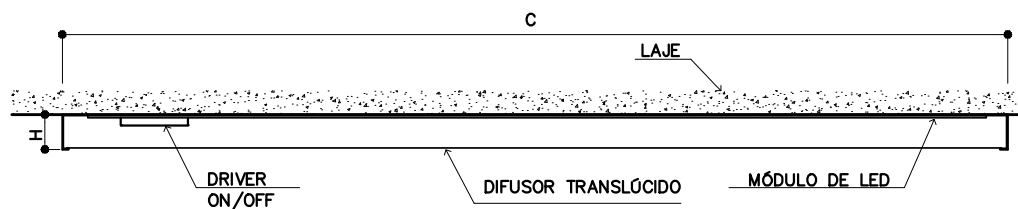
IL-90 LUMINÁRIA LED INTEGRADA CORTE LONGITUDINAL S/ESC.
