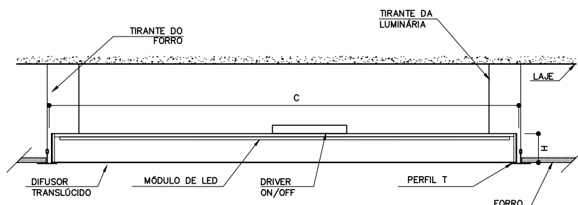
VISTA LONGITUDINAL
