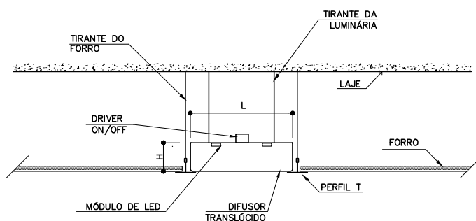
CORTE TRANSVERSAL
