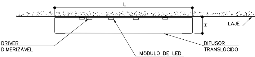
CORTE TRANSVERSAL S/ESC.
