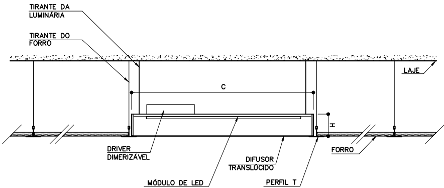
VISTA LONGITUDINAL S/ESC.
