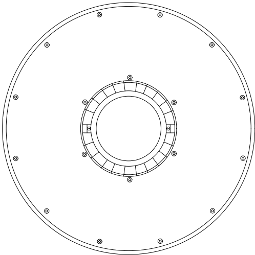
OPÇÃO 2: VISTA INFERIOR S/ESC.
