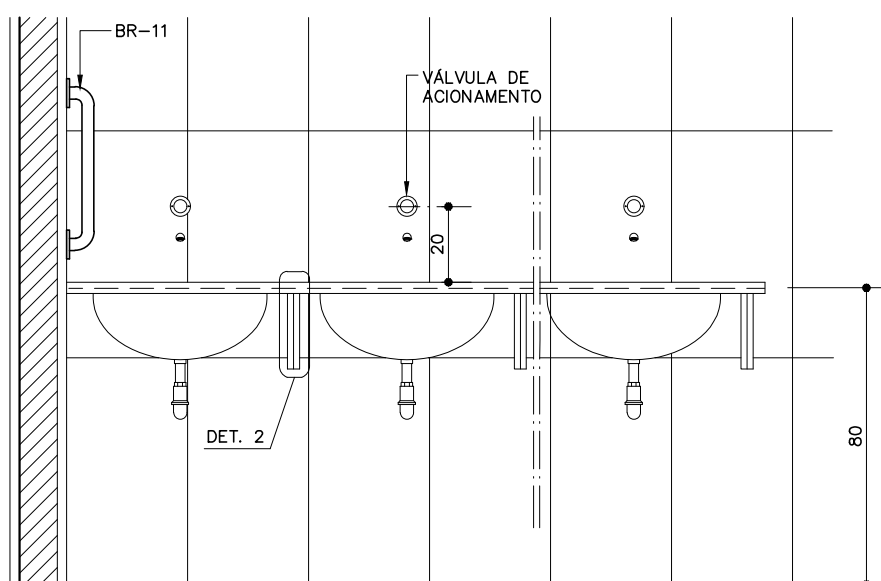
VISTA 1
