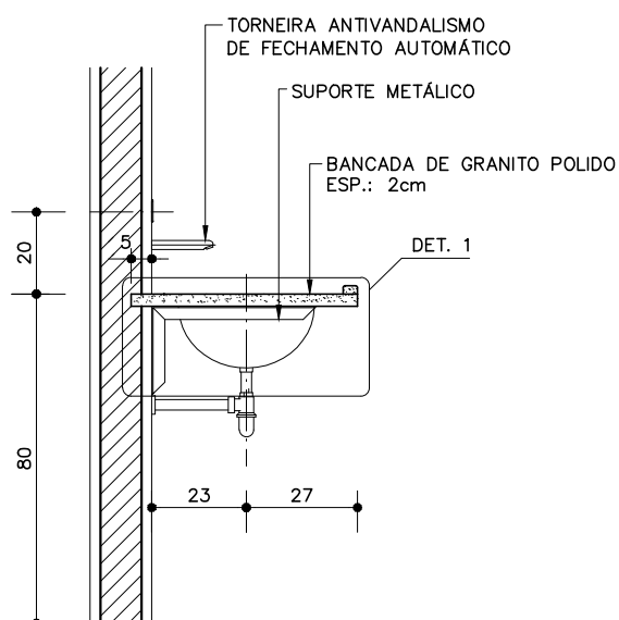
CORTE AA
