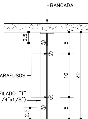
DETALHE 2
