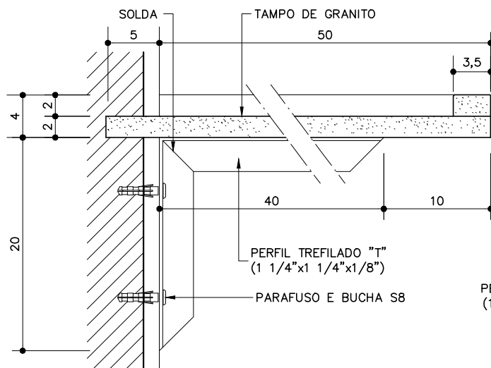
DETALHE 1
