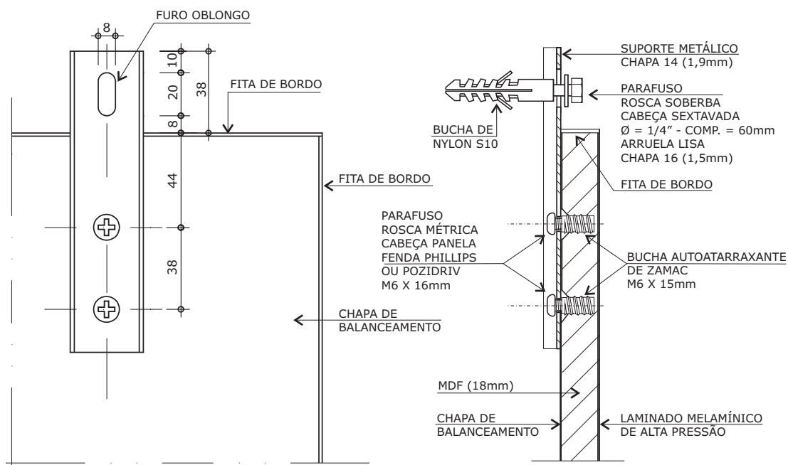
VISTA POSTERIOR
