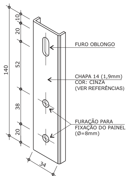
SUORTE METÁLICO
