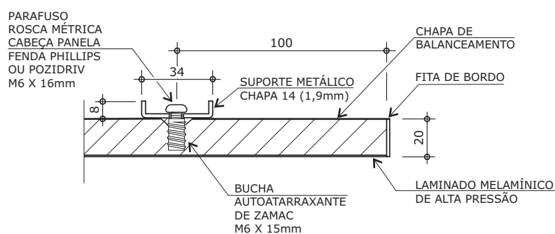
CORTE LONGITUDINAL
