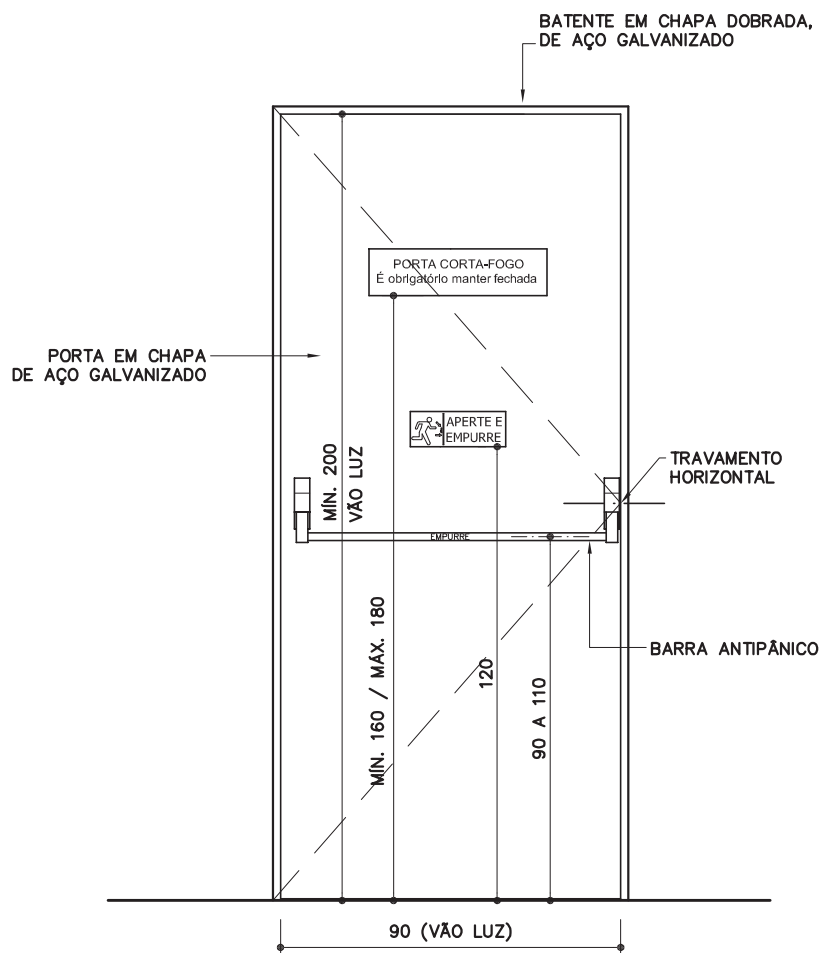
ELEVAÇÃO 1 ESC. 1: 20
