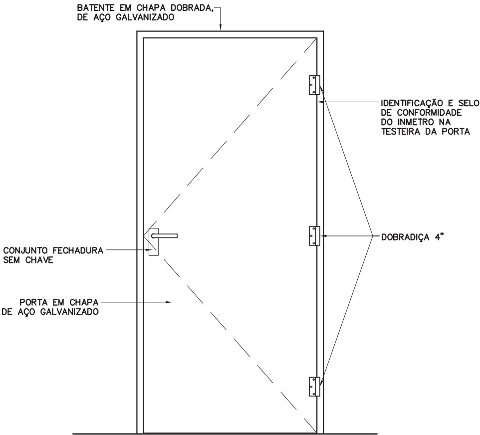
ELEVAÇÃO 2 ESC. 1: 20
