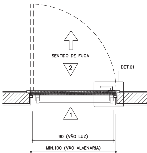
PLANTA ESC. 1: 20
