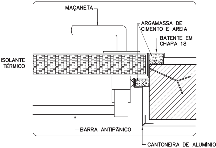
DETALHE 01 ESC. 1: 5
