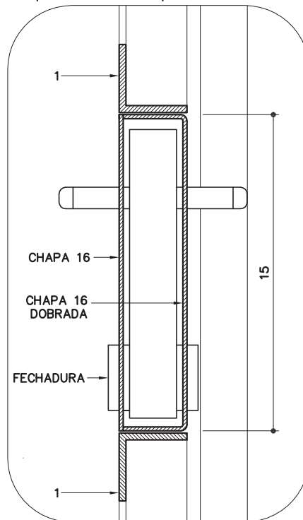
DET. 3 ESC. 1:2.5
