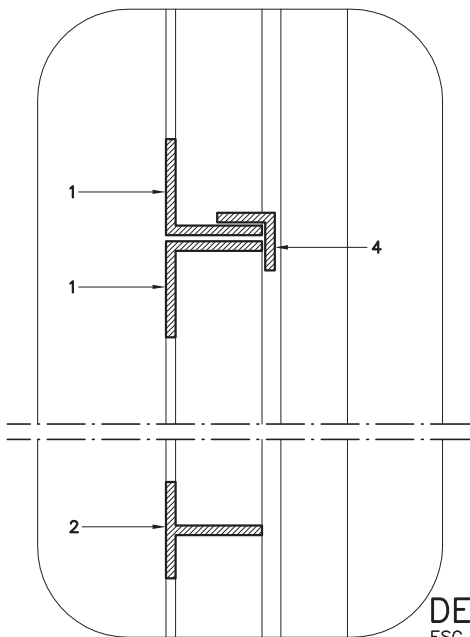
DET. 3 ESC. 1:2.5
