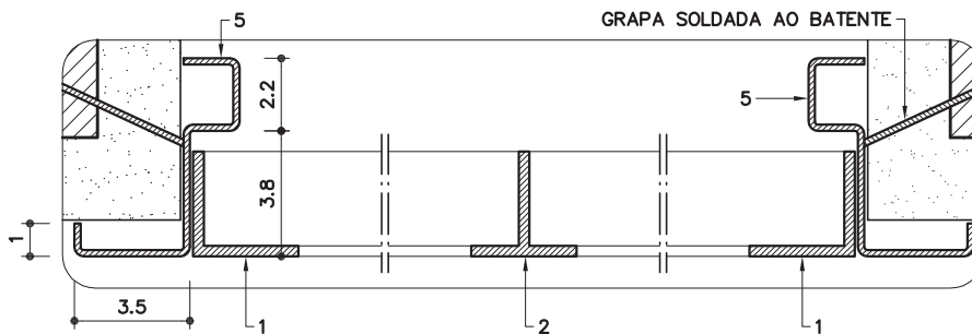
DET. 1 ESC. 1:2.5
