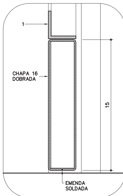
DET. 4 ESC. 1:2.5
