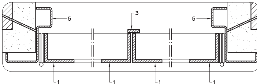
DET. 2 ESC. 1:2.5
