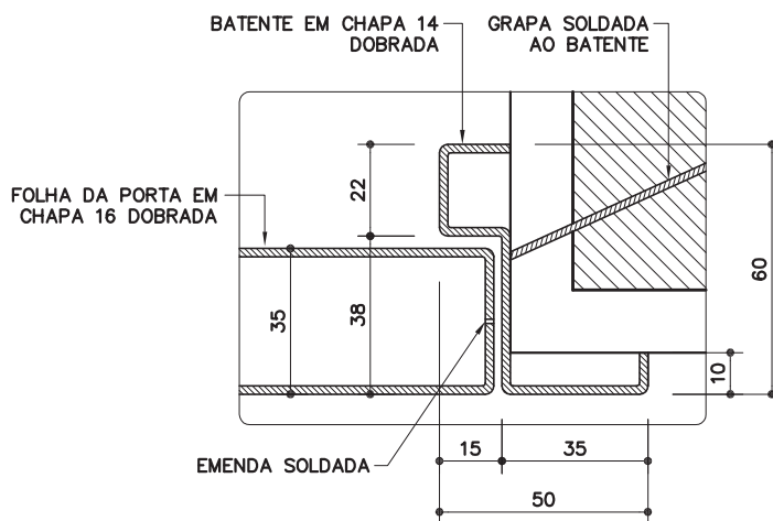
DETALHE DO BATENTE
