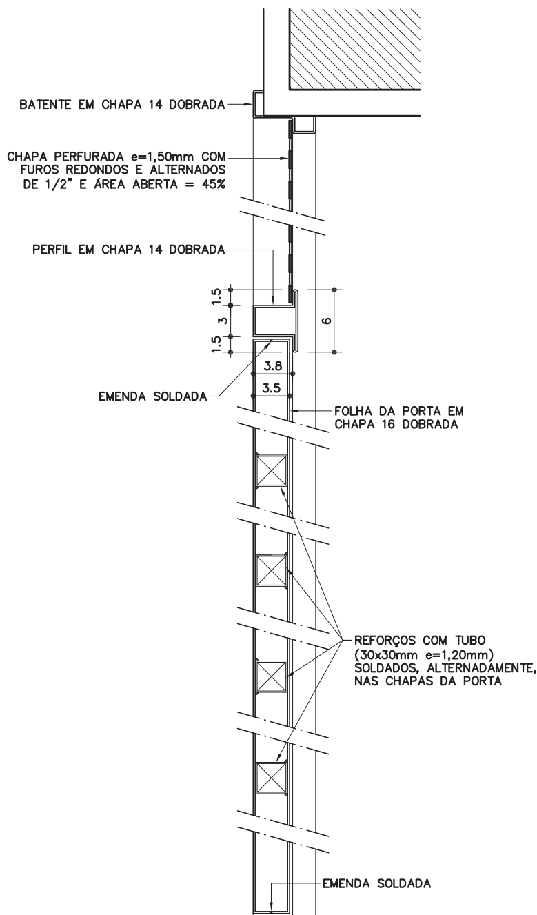
DETALHE 02
