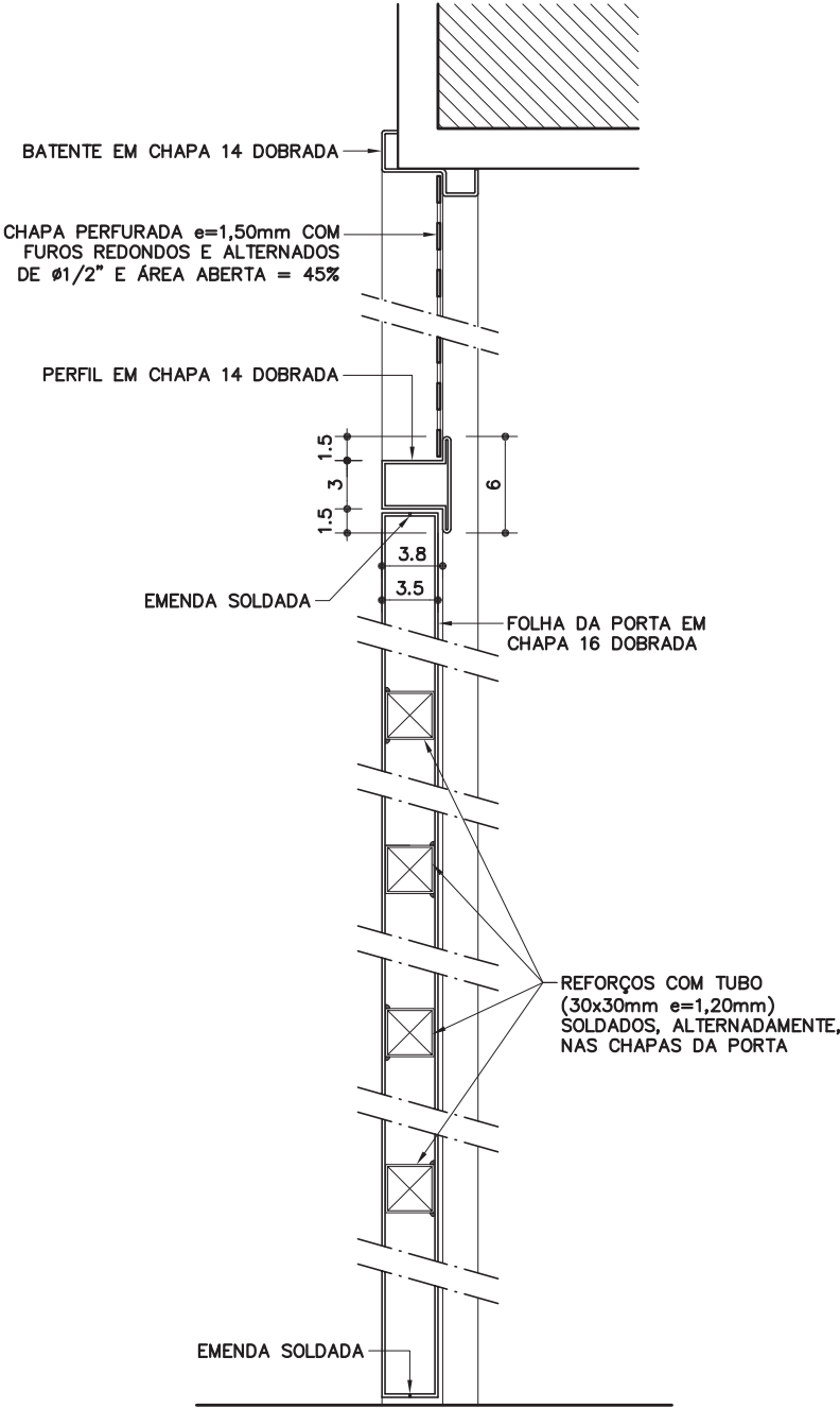
DETALHE 02 ESC. 1:5
