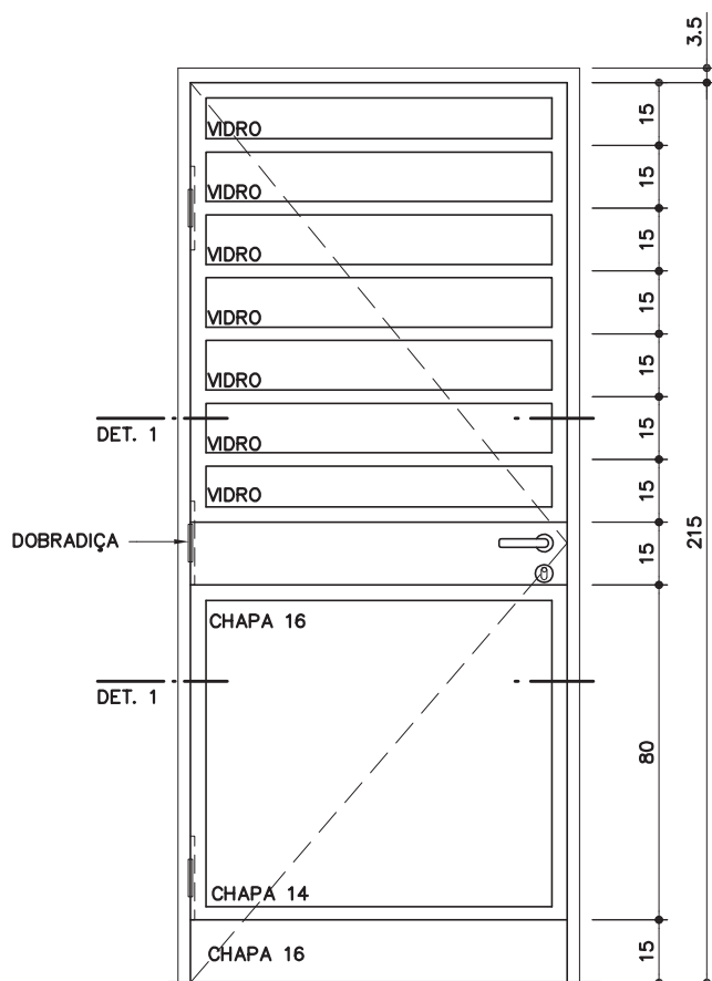
VISTA ESC. 1:20
