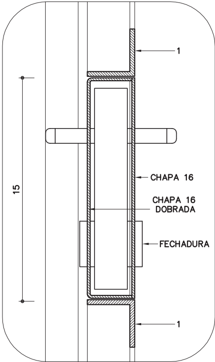
DET. 3 ESC. 1: 2.5
