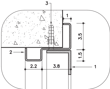
DET. 2 ESC. 1: 2.5
