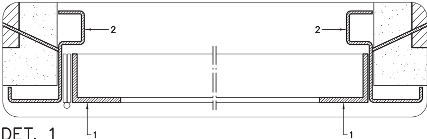
DET. 1 ESC. 1: 2.5
