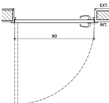
PLANTA ESC. 1:20
