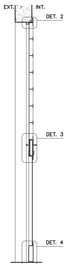
CORTE ESC. 1:20
