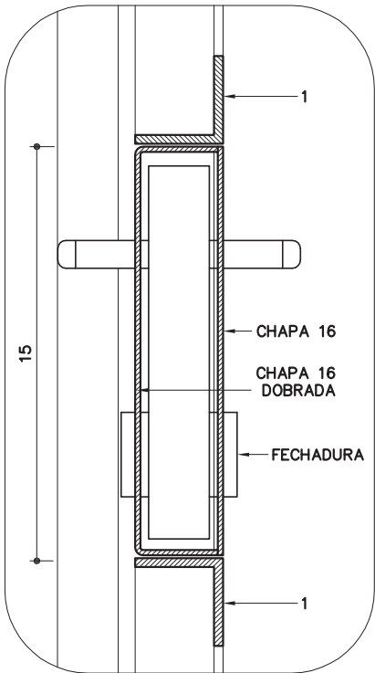
DET. 5 ESC. 1:2.5
