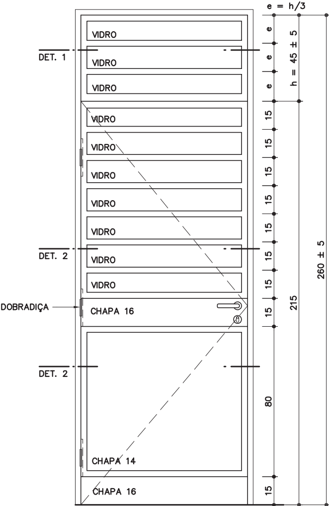
VISTA ESC. 1:20
