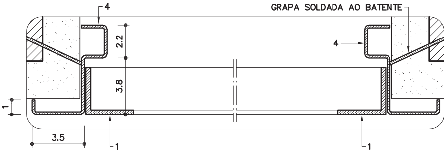
DET. 1 ESC. 1:2.5
