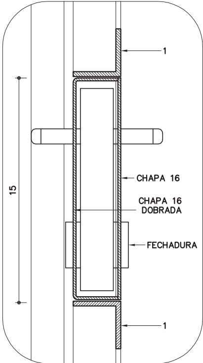
DET. 5 ESC. 1:2.5
