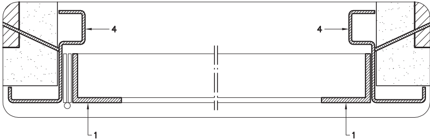
DET. 2 ESC. 1:2.5
