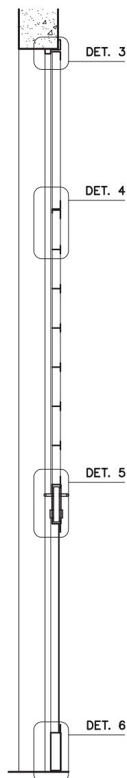
CORTE ESC. 1:20
