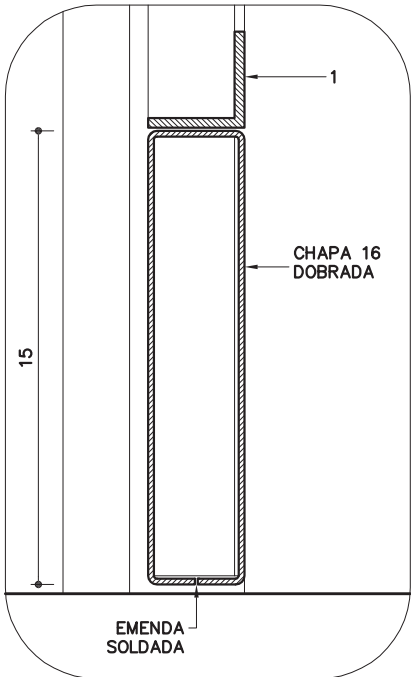
DET. 6 ESC. 1:2.5
