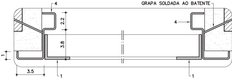
DET. 1 ESC. 1:2.5
