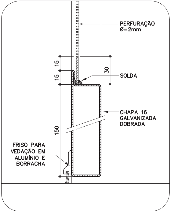
DET. 4 ESC. 1:2.5 MEDIDAS EM mm
