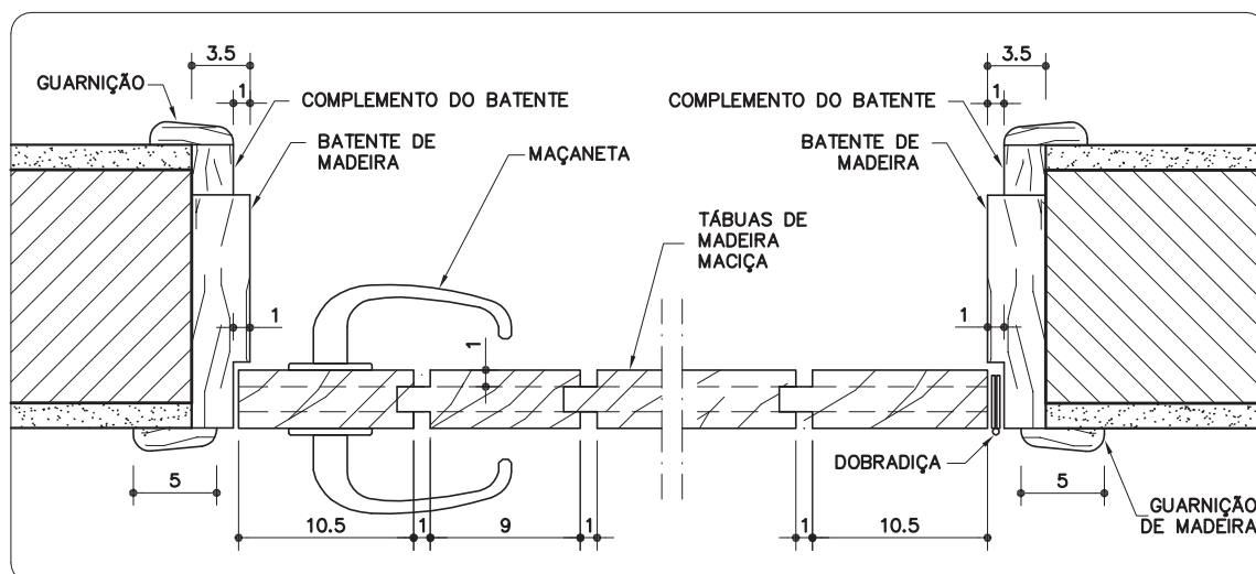
DETALHE 1 ESC. 1:5
