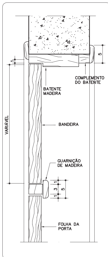
DETALHE 4 BATENTE DE MADEIRA ESC. 1:5
