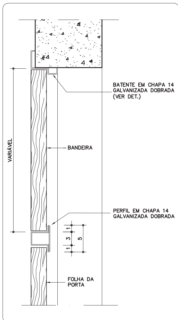
DETALHE 3 BATENTE METÁLICO ESC. 1:5
