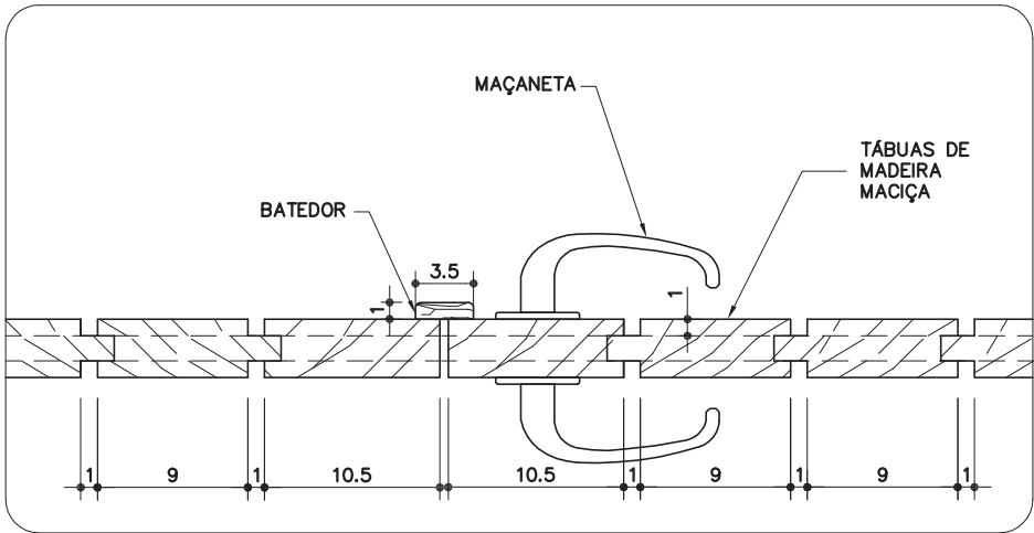
DETALHE 2 ESC. 1: 5
