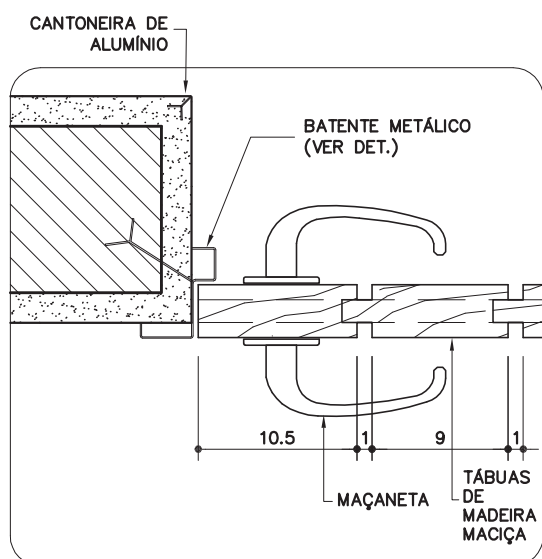
DETALHE 1 ESC. 1:5
