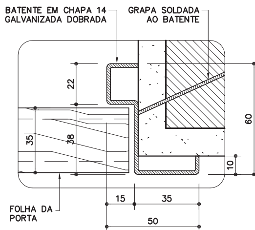
DETALHE DO BATENTE METÁLICO
