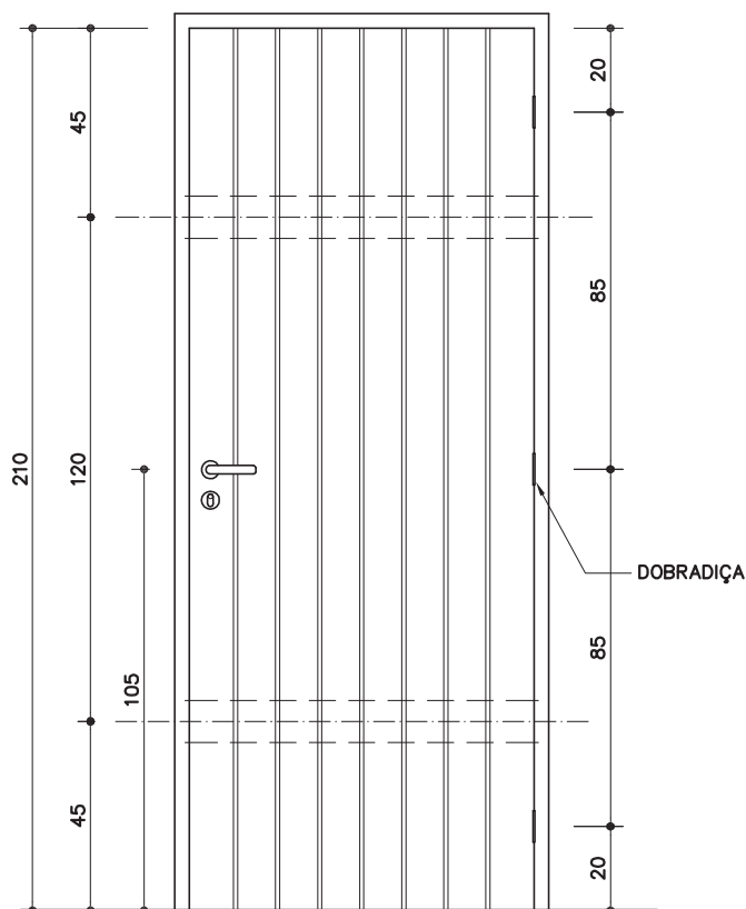
VISTA ESC. 1:20
