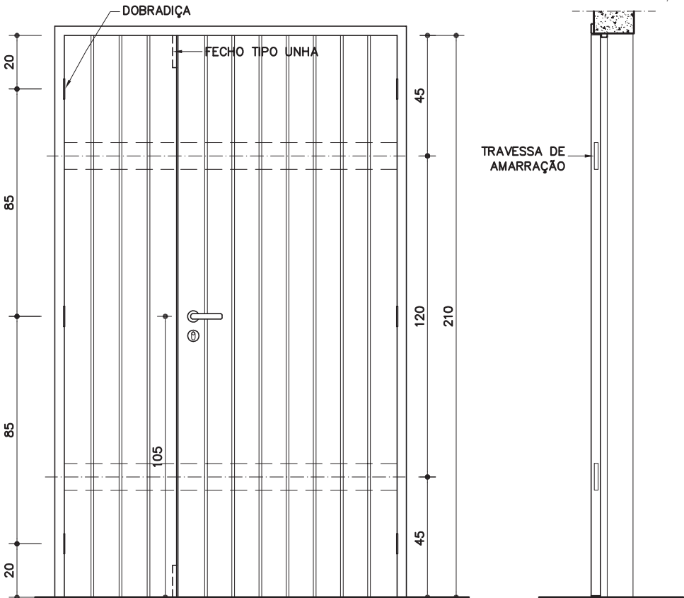
VISTA ESC. 1: 20
