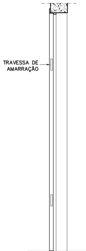
CORTE ESC. 1:20
