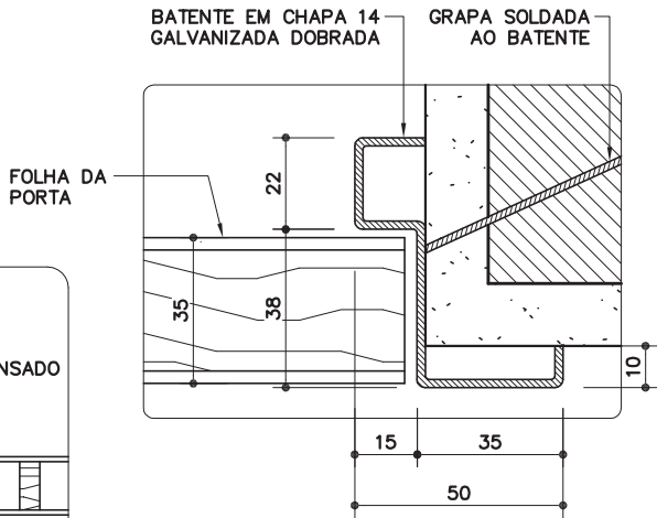
DETALHE DO BATENTE METÁLICO
