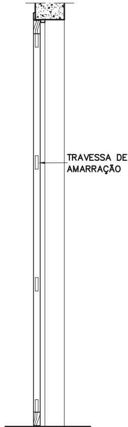
CORTE ESC. 1: 20
