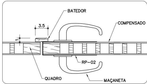
DETALHE 2 ESC. 1: 5
