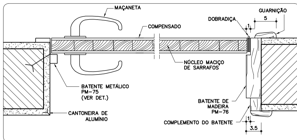
DETALHE 1
