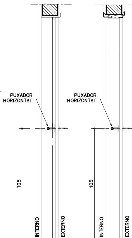
CORTE
