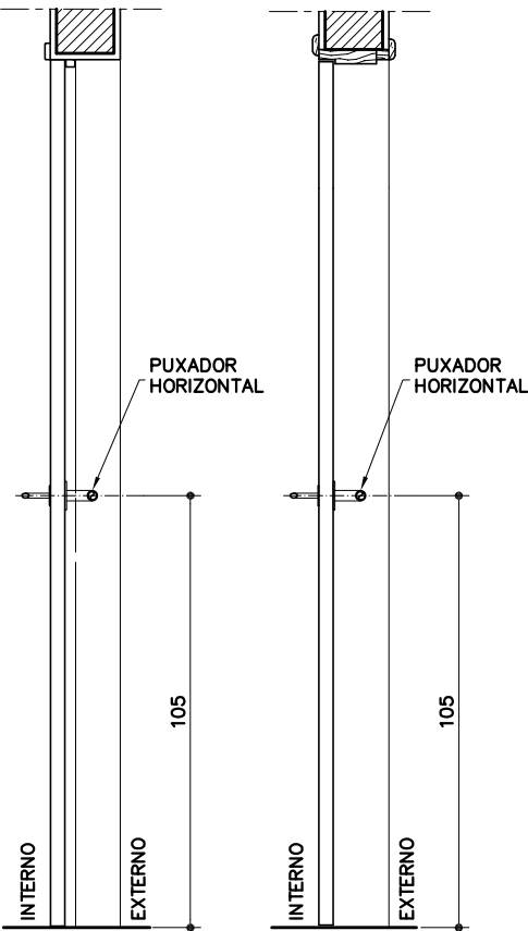
CORTE BB
