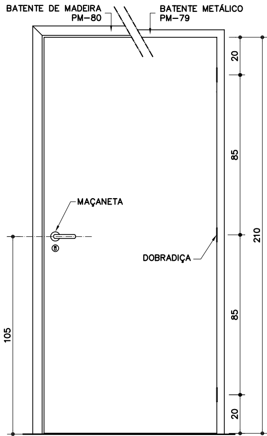
VISTA 4 – INTERNA
