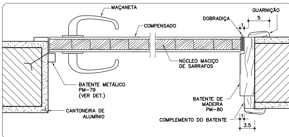
DETALHE 1
