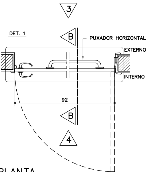
PLANTA
