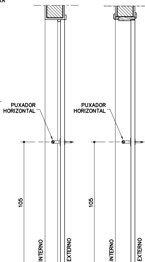
CORTE AA
