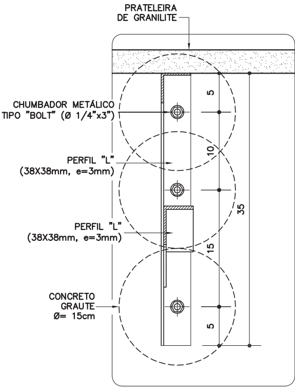
DETALHE 2 ESC. 1:5
