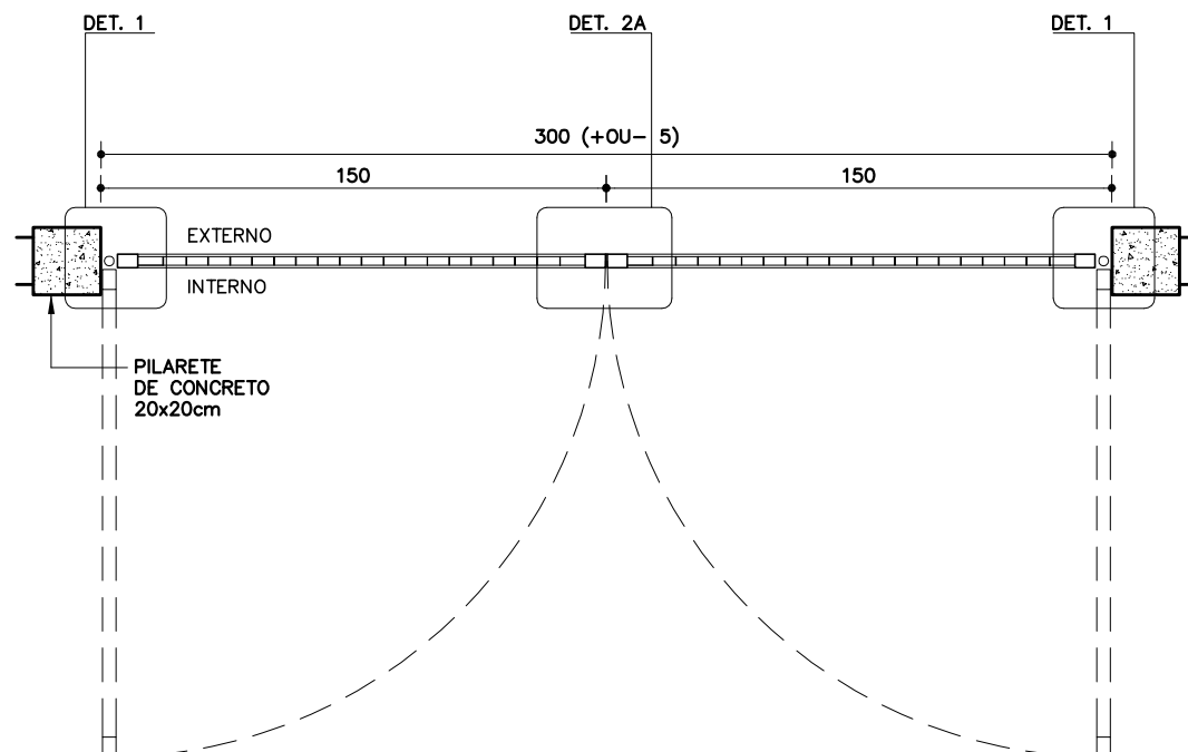
PLANTA PT-31
