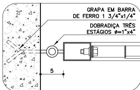
DETALHE 1 ESC. 1:5
