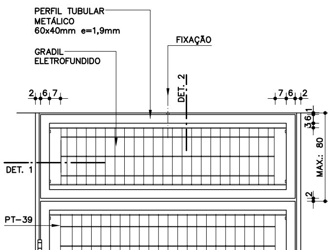
VISTA INTERNA PT-40
