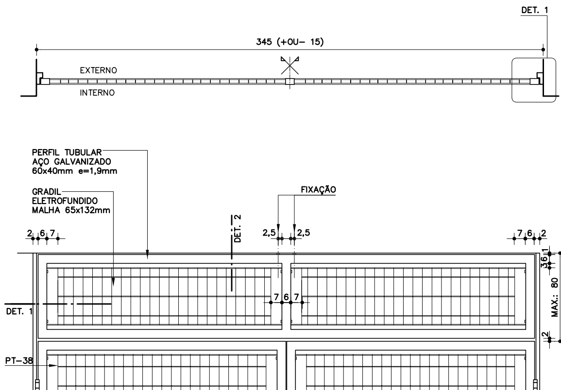
VISTA INTERNA PT-40
