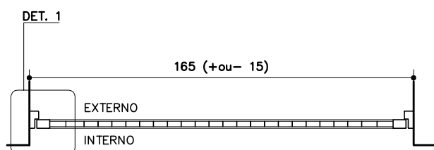
PLANTA PT-40
